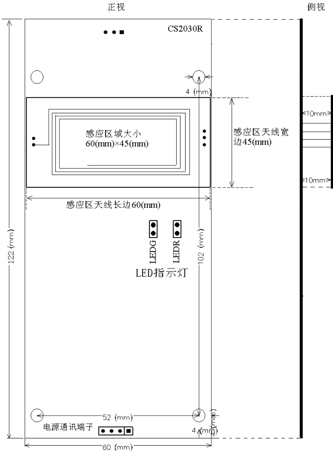
IC卡读写板相关尺寸示意图
