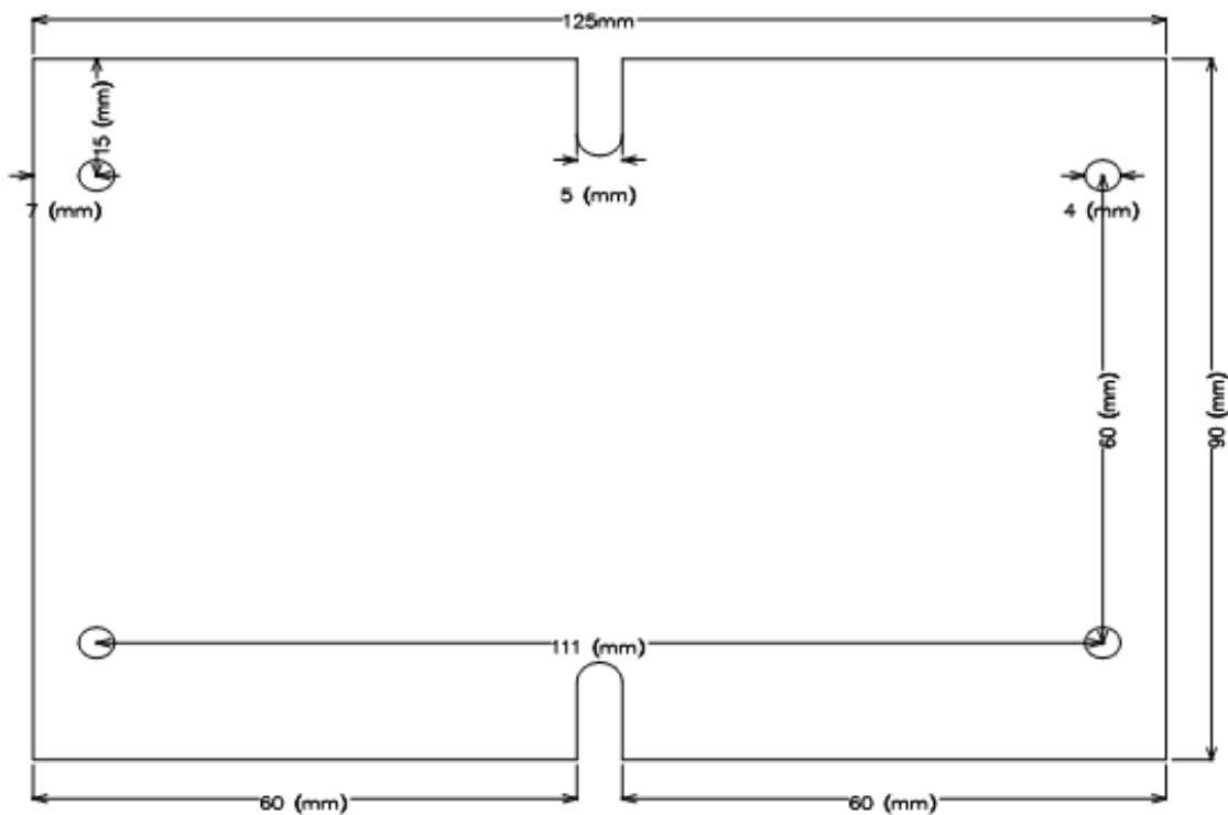
IC卡控制器的安装衬板示意图
